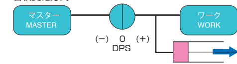
容積変化方式 Volumetric change method
