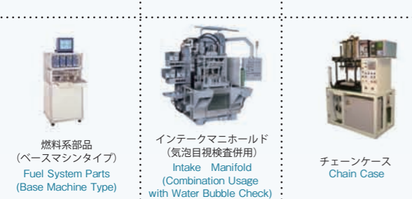
キャニスター Canister EGR クーラー ASSY EGR COOLER ASSY 発電機インテークマニホールド GENSET INTAKE MANIFOLD
