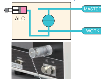
容積変化方式 Volumetric change method
