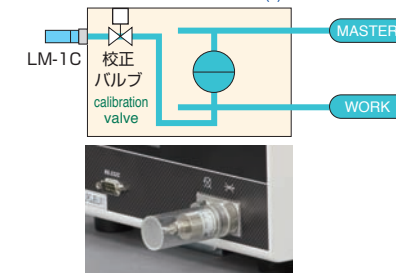
漏れ基準方式 Leak reference method
